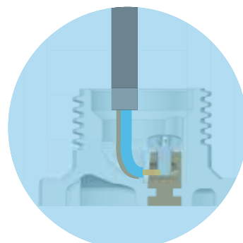
Connessione semplificata con raccordi incorporati.
